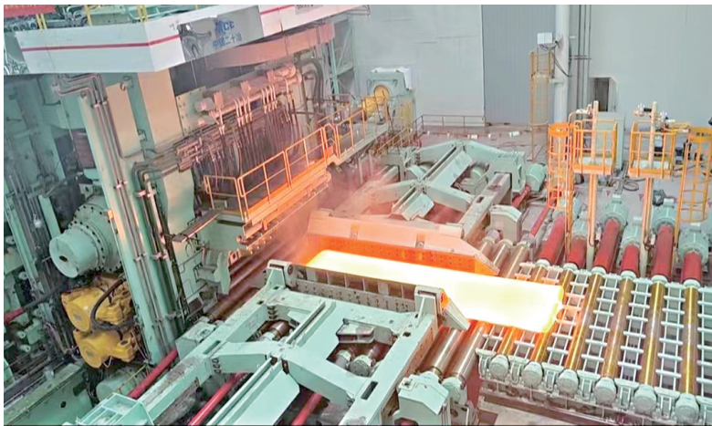
图为主轧线热负荷试车场景。
